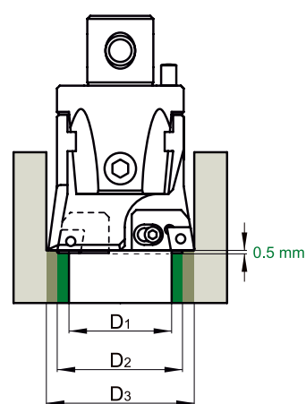
Stupňovité vyvrtávání
